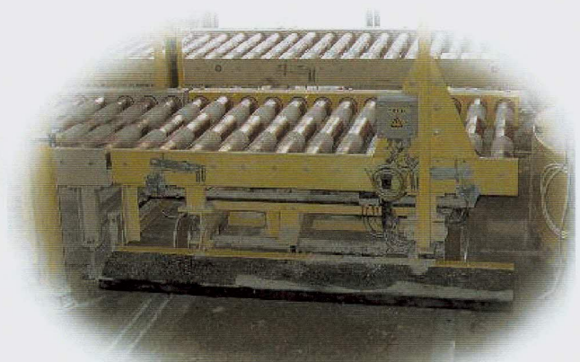
Palettenumsetzwagen Pallet-transfer-shuttle
