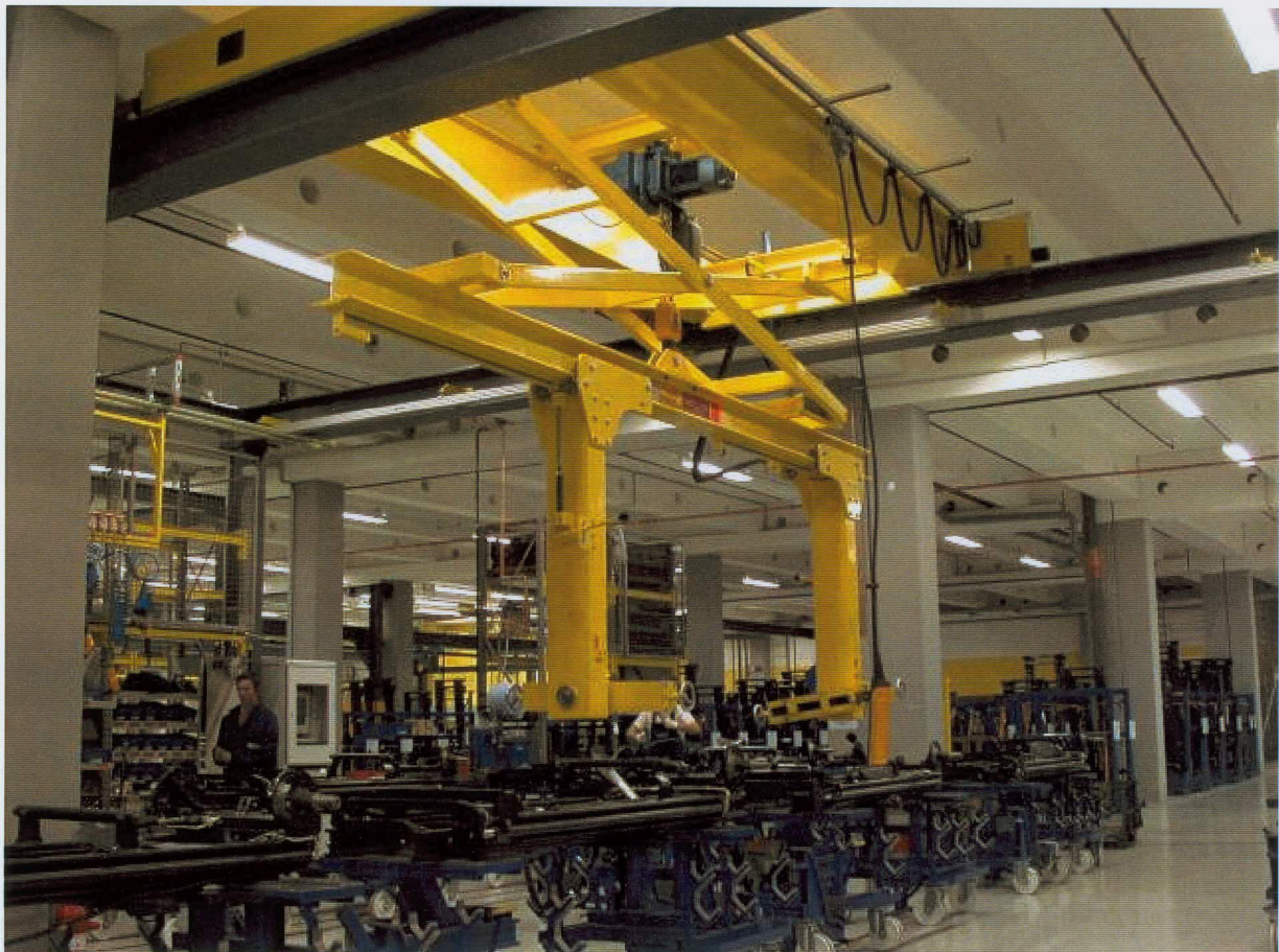
Handlingseinrichtung als Mehrplatzsystem in der Gabelstaplerfertigung Mobile jigs and assembly aids
